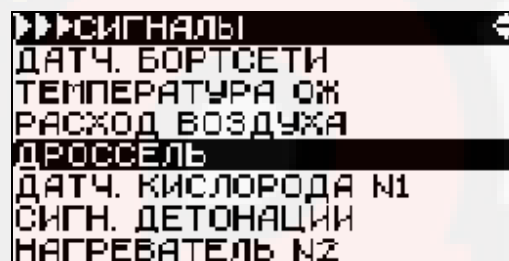
Рис. 14 Меню СИГНАЛЫ
