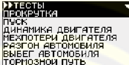
Рис. 25 Меню ТЕСТЫ
