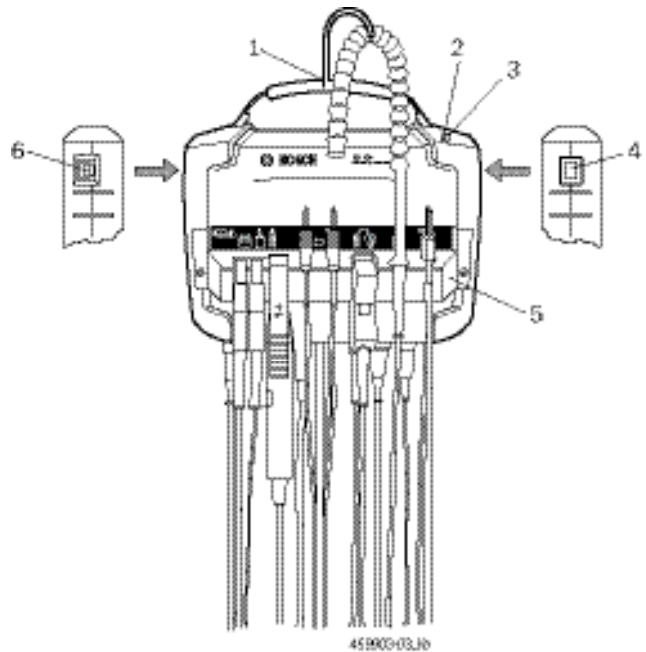
Fig. 1: Вид спереди FSA 500
