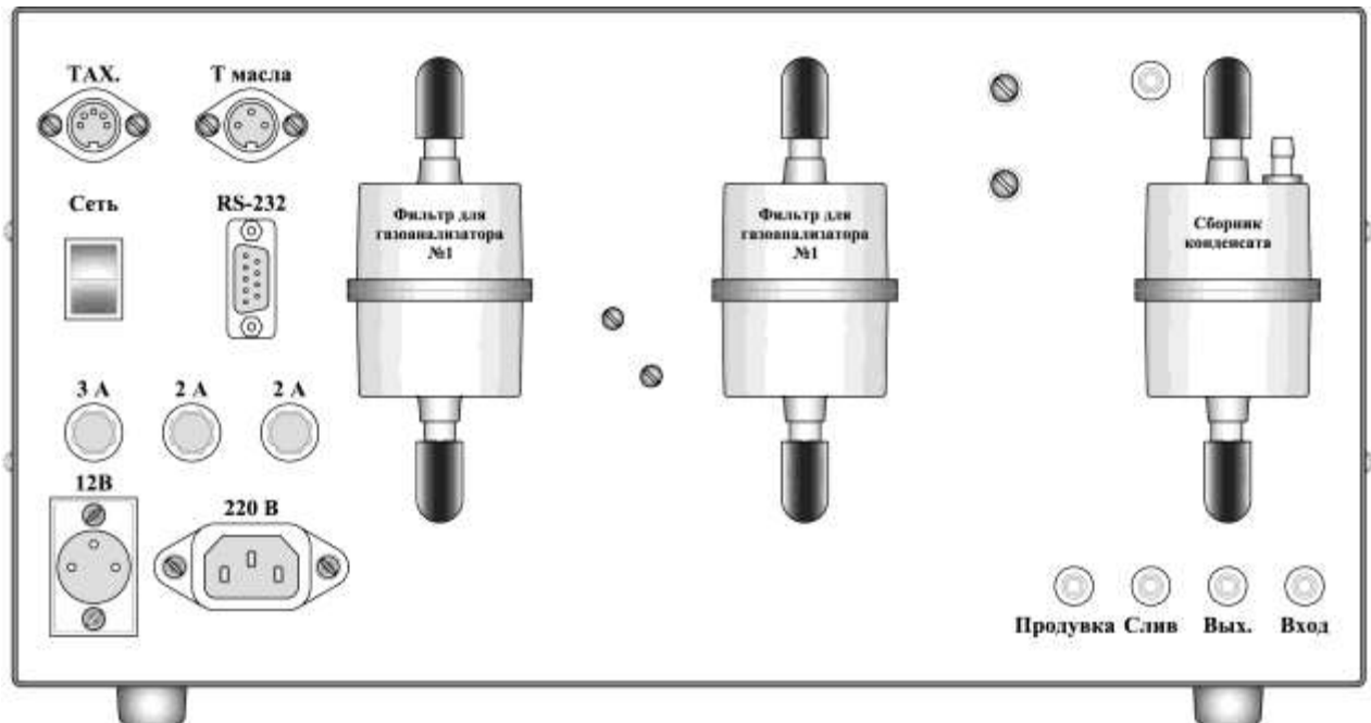
Рис.Г.2.Вид сзади
