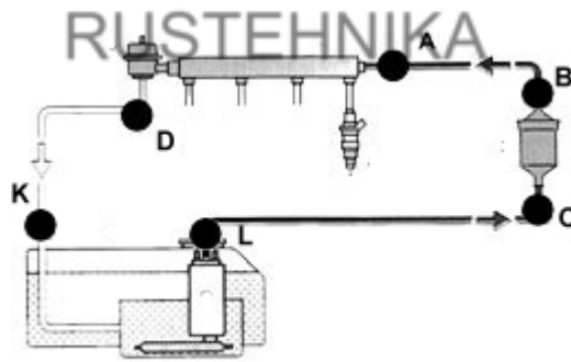
Система L- JETRONIC/ MOTRONIC с топливным электронасосом, установленном в топливном баке
