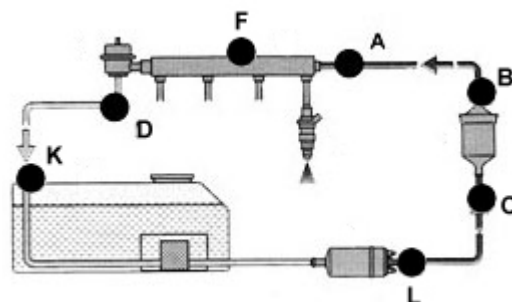
Система L- JETRONIC/ MOTRONIC с топливным электронасосом, установленном в топливопроводе последовательно с топливным баком
