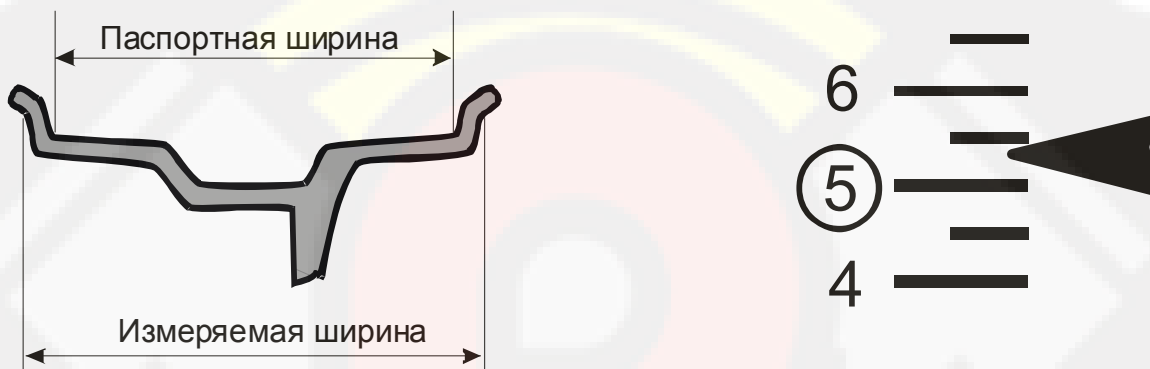
а – паспортная и измеряемая ширина диска б – ближайшее меньшее значение 5 дюймов (5") Рисунок 2.9
