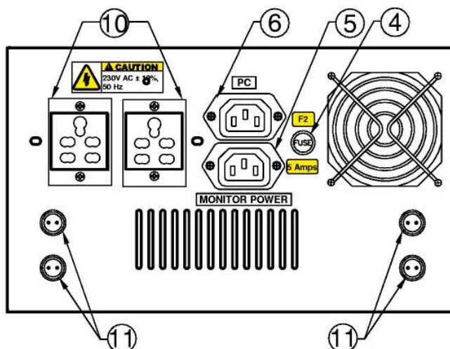
РИС. 26 Интерфейсный блок – Вид спереди (внутри мобильного шкафа)
