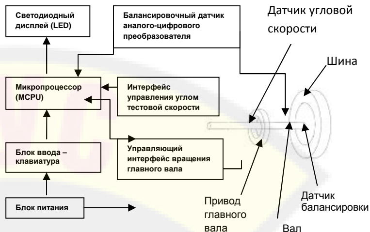
РИС. 3 ПРИНЦИП РАБОТЫ БАЛАНСИРОВОЧНОГО СТАНКА 4524Е
