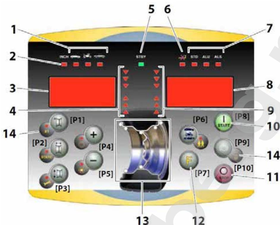
Рис. 1 – Панель управления
