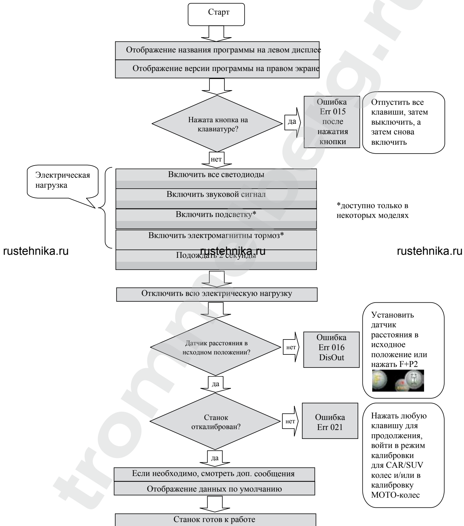
Диаграмма программ при запуске станка
